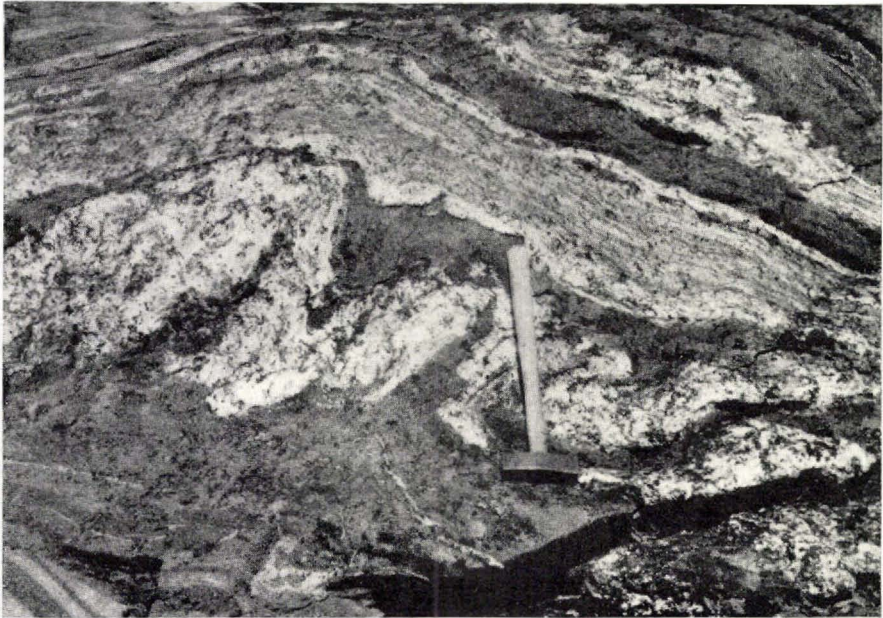
Fig. 54: Intrusion ptygmatisique, selon la définition de G. WILSON (1952), dans le gneiss rubané de la région au S de Puiátup tasé. Photo M. BURRI.
