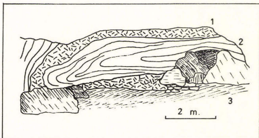
Fig. 52: S de Puiátup tasè. Dans des gneiss rubanés (2), plis couché se rapportant à la première phase de plissement et nettement souligné par une pegmatite syn-cinématique (1). Le premier plan est recouvert de débris quaternaires (3). Dessin d'après photo.
