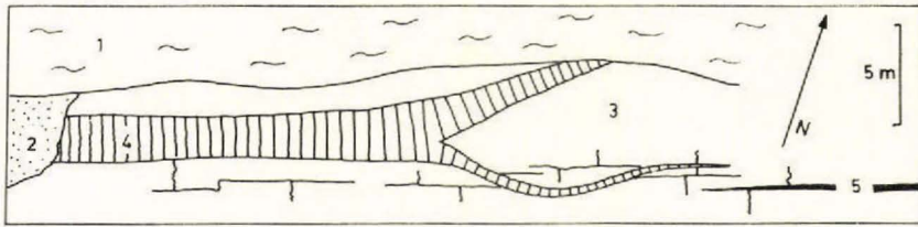
Fig. 42: Côte S de Sermiligårssuk, en face de l'île, visible à marée basse seulement.
