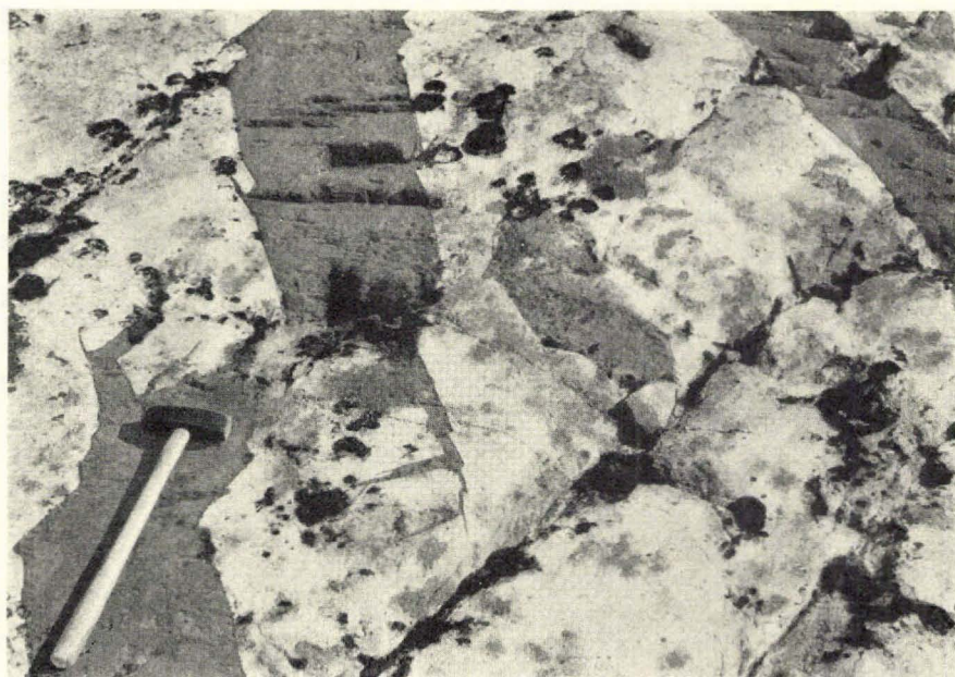
Fig. 36: Entre le Gaffelso et de pt. 880. Deux petits filons lamprophyriques faisant partie d'un essaim de filons parallèles. On remarque très bien les relations entre les diaclases du gneiss et la tectonique d'intrusion du filon (cf. S. KAITARO, 1952 et C. E. WEGMANN, 1938, p. 85). Photo M. WEIDMANN.
