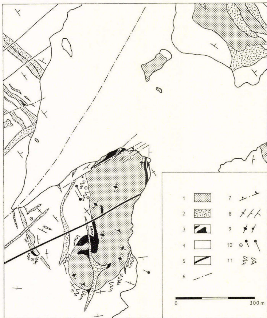
Fig. 15: Carte schématique, d'après les travaux de terrain, d'une partie des ultramafites (sills, lentilles et massifs) de la région du lac 510. (Siksakso).
