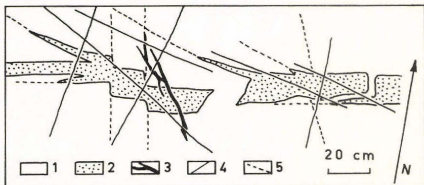
Fig. 48: 1 km. à l'W du lac 665. Petite apophyse d'un BDo.
