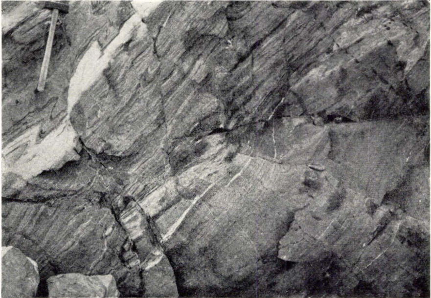
Fig. 2: Côte S de Sermiligårssuk fjord, au N du pt 1018. Schistes pélitiques finement lités, microplissés et coupés par quelques cassures verticales; on note une mince couche quartzofeldspathique claire sur la gauche. Photo M. WEIDMANN.
