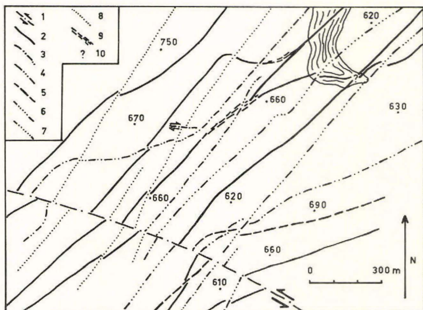
Fig. 26: Région située entre Qaersutsiaq et le pt. 690. Cette zone est caractérisée par un faisceau formé par de très nombreux filons d'âges différents. Les recouvrements sont courants et très bien visibles sur le terrain.
