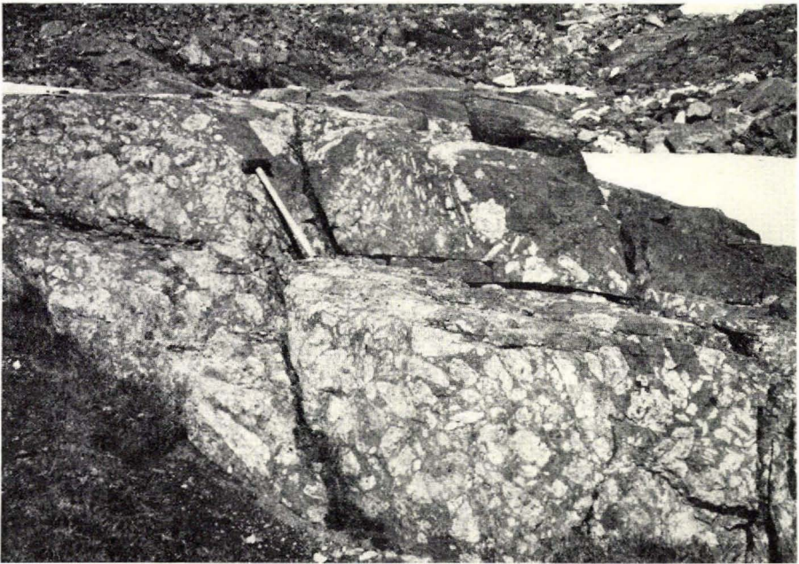
Fig. 46: W de Bikuben. Faciès très grossièrement porphyrique et xénolitique à la bordure NW du BD. Il faut noter le contact très brusque avec une apophyse sombre, non porphyrique, finement cristallisée, qui est émise par le corps principal du filon et qui coupe la masse porphyrique; c'est là un indice d'intrusion multiple, prolongée dans le temps. Photo M. WEIDMANN.
