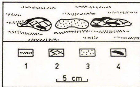
Fig. 27: NW du Gaffelso.
