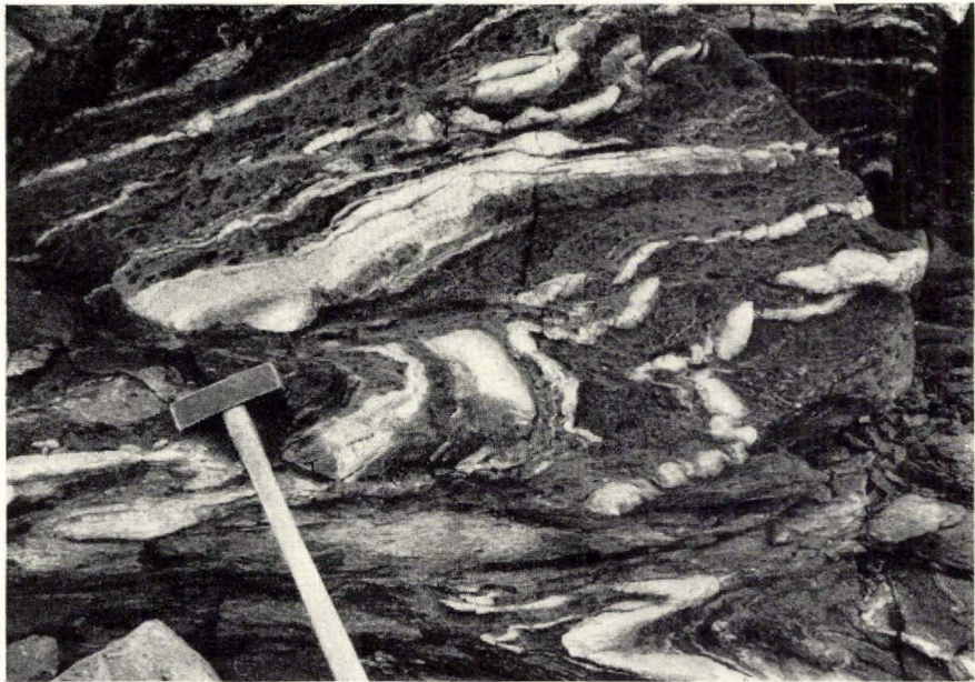
Fig. 4: SE de Lysefjeld. Fragment de schiste en voie de gneissification, compris entre des pegmatites; les nombreux lits quartzofeldspathiques sont ici plissés, boudinés, cassés et forment parfois des «quartz-rods» (G. WILSON, 1953); le contact entre les lits acides et la trame basique est moins tranché que les contacts schiste-pegmatite de la fig. 3. Photo M. WEIDMANN.
