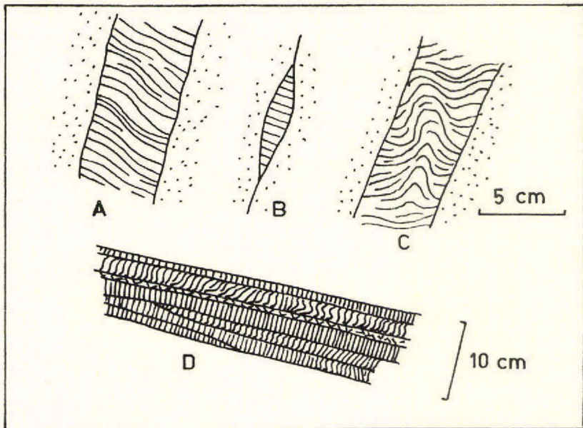
Fig. 17: Massif 510. Quatre types de remplissage de diaclase:
