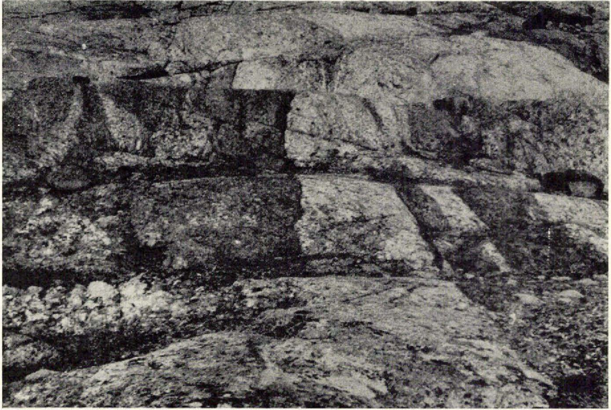
Fig. 9: Pt. 880, N du Gaffelsø. Gneiss à trainées basiques; masses quartzofeldspathiques différenciées riche en muscovite et reliques basiques à chlorite et épidote. Le contact est soit tranché, soit diffus. Photo M. WEIDMANN.
