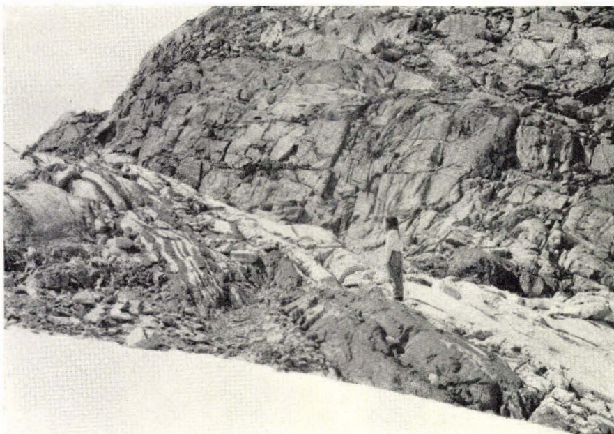
Fig. 50: 1 km. à l'W du lac 665. Un BDo de 25 m. émet une apophyse large de 3 m. qui n'est pratiquement pas ramifiée là où se tient le personnage qui donne l'échelle; ensuite le filon se transforme très rapidement en une quinzaine d'intrusions parallèles qui se suivent sur 20 m. environ avant de disparaître. Photo M. WEIDMANN.
