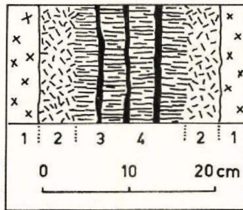
Fig. 37: Pt. 685, N du Gaffelsø. Coupe d'un petit JD montrant une texture due semble-t-il, à une activité hydrothermale prolongée et postérieure à la cristallisation du magma aux éponites du filon.
