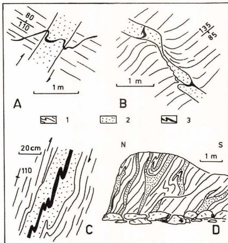
Fig. 31: Exemples de déformations lors du métamorphisme sanerutien. Région du massif septentrional des granites de Tigssaluk.
