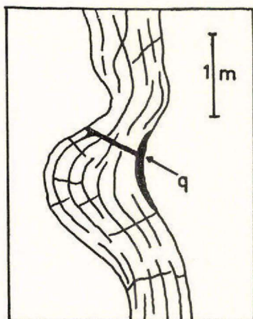
Fig. 25: NW du pt. 640, NW du Gaffelsø. Exemple d'AD localement sinueuse et étranglée. Les diaclases longitudinales sont les plus nombreuses et épousent la forme du filon. Veines de quartz (q) le long d'une éponte et dans une diaclase transversale. Croquis d'après photo.
