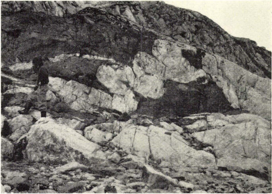
Fig. 11: E du pt. 1018. Dans le gneiss agmatitique, grosse pegmatite discordante à plis ptygmaticques, comprise entre deux corps pegmatitiques plus ou moins concordants qui enserrant une relique de schistes basiques. Photo M. WEIDMANN.
