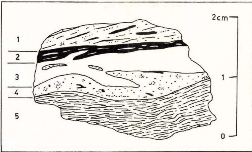
Fig. 41: Echantillon 38061, pris sur le contact filon-roche encaissante (voir fig. 42) dans un trachyte du type sodique, côte S de Sermiligårssuk fjord, en face de l'île. Le filon s'est mis en place dans un gneiss agmatitique albito-chloriteux, en voie de granitisation et très mylonitisé.
