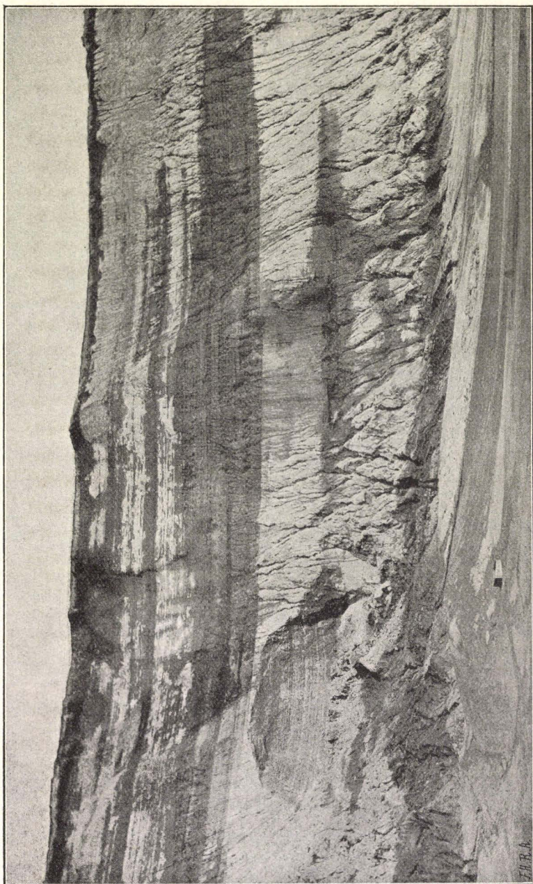
Fig. 12. Klinten N. for Grotten. Profilets Højde c. 27 M. Sml. Teksten S. 196.
