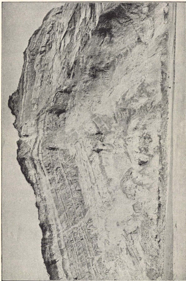
Fig. 2. Umiddelbart Syd for Søndre Stensue Rende. Profilets Højde ca. 40 M. Sml. Teksten S. 67.
