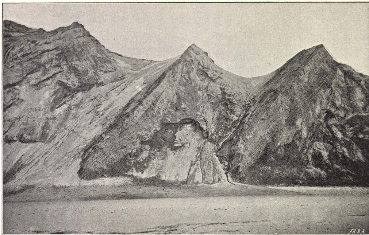
Fig. 3. Nord for Søndre Stenstue Rende. Profilets Højde 25—30 M. Sml. Teksten S. 70.
