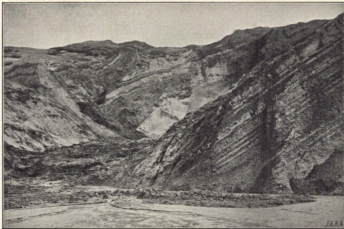
Fig. 6. Søndre Stenstue Rende. Profilets Højde ca. 40 M. Sml. Teksten S. 75.
