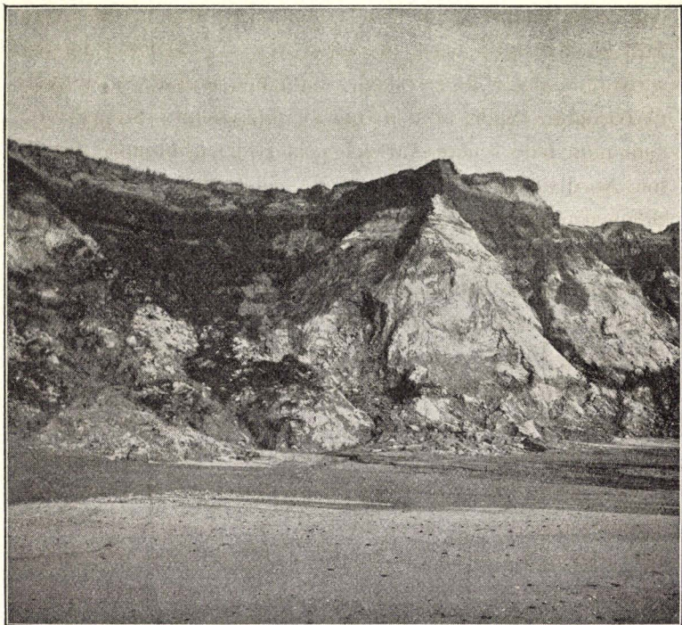
Fig. 13. Martørv Bakker. Klintens Højde c. 30 M. Sml. Teksten S. 235.
