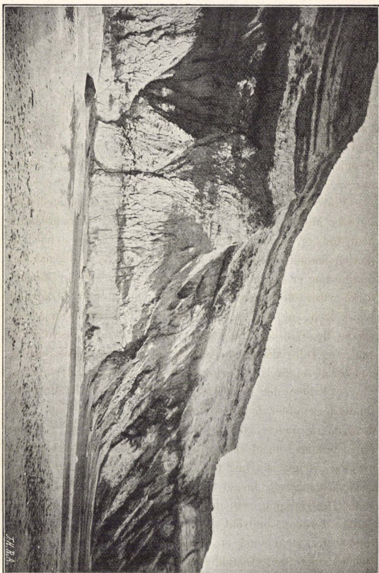
Fig. 10. Profil mellem Martøv Bakker og Stensnes. Sml. Teksten S. 123.
