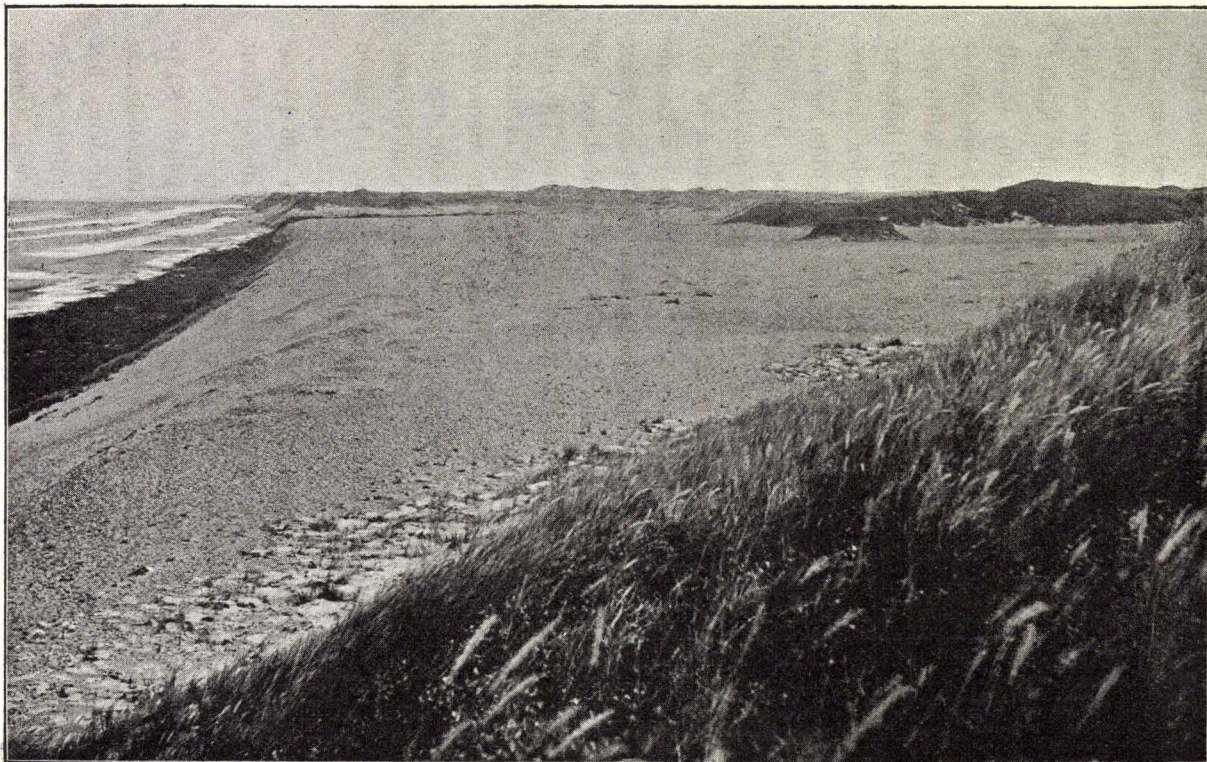
Fig. 15. Stensletten Raabjerg Stene. Sml. Teksten S. 270.
