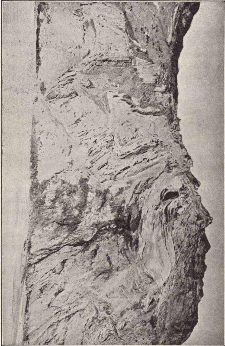
Fig. 9. Syd for Nørre grønne Rende. Profillets Højde ca. 35 M. Sm. Teksten S. 91.
