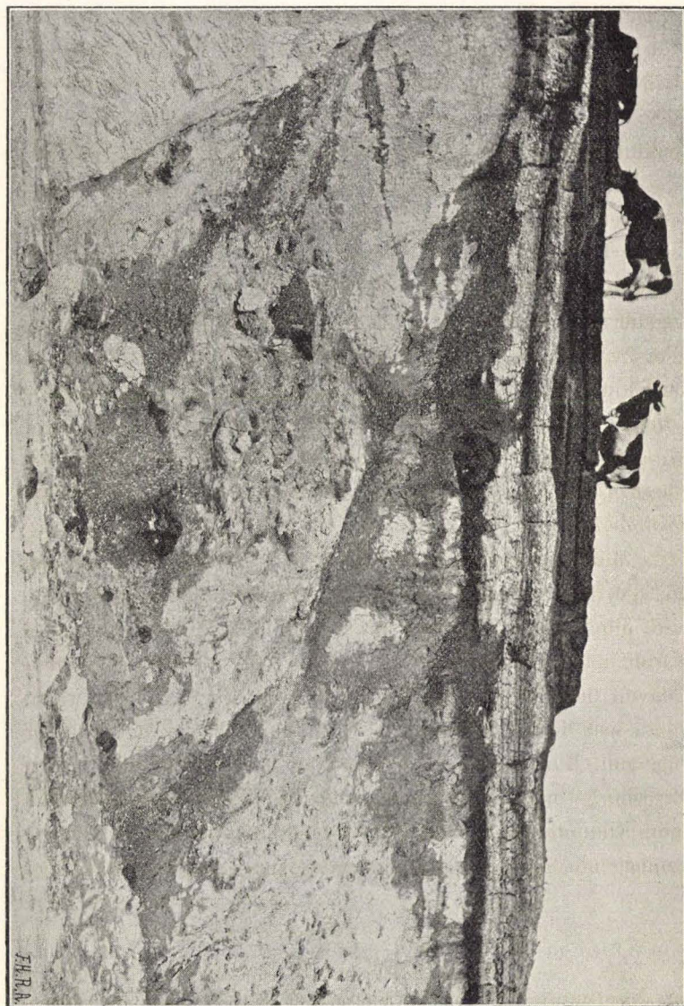
Fig. 16. Nordsiden af Kloften ved Kodals Rende.
