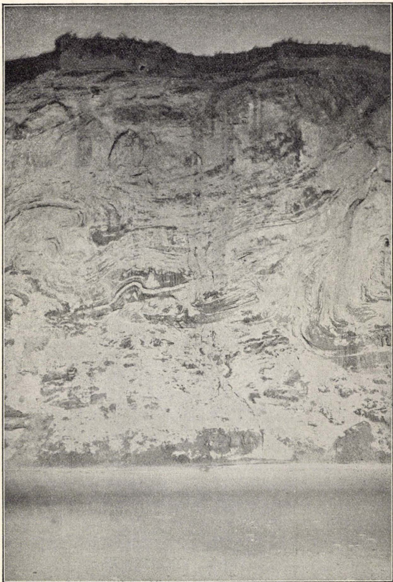
Fig. 7. Syd for Stensnæs. Profilets Højde ca. 33 M. Sml. Teksten S. 75.
