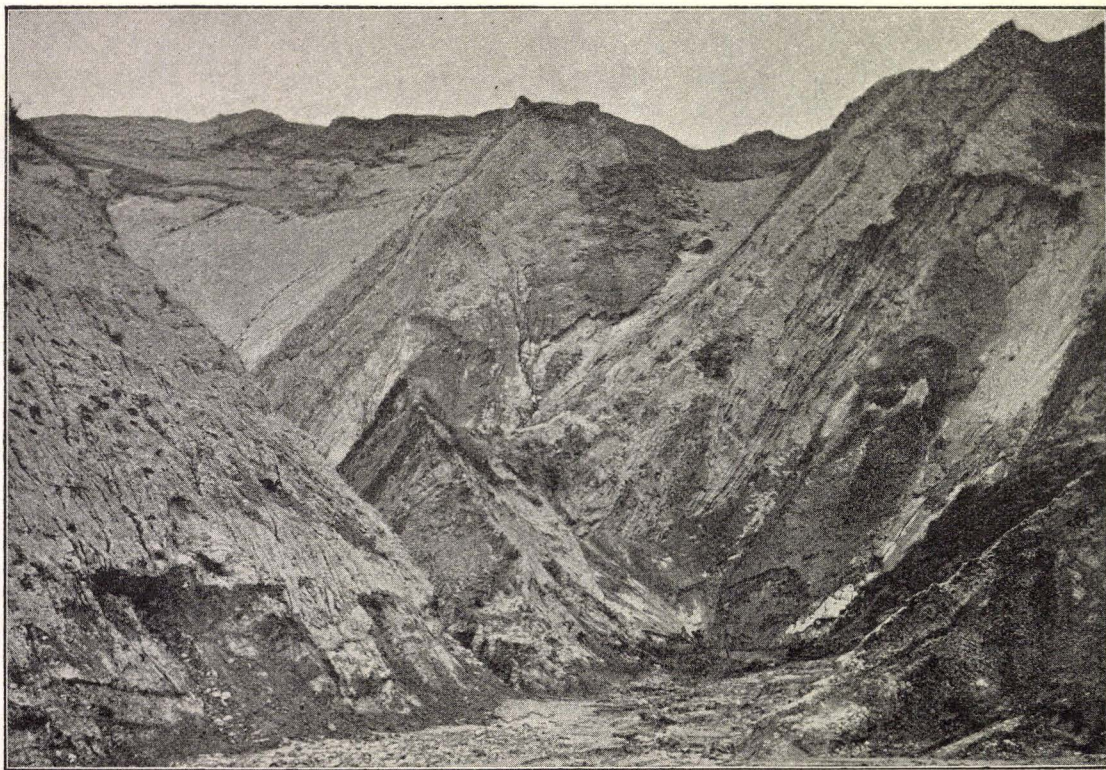
Fig. 5. Nørre grønne Rende. Profilets Højde ca. 50 M. Sml. Teksten S. 75.
