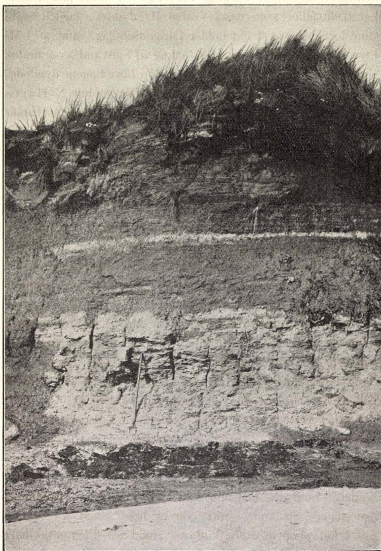
Fig. 14. Munden af Klostergrøft. Tørv dækket af Saltvandsler og Flyvesand. Profilets Højde 4—5 Meter.
