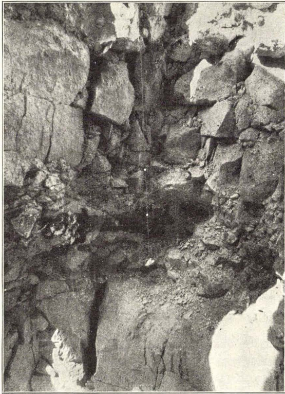
Fig. 4. Spalte i den faste Kalk i en Skrænt med »Faarestier«. Lodsnoeren angiver Vertikalen og Afstanden mellem Knuderne paa Snoren er 10 cm. Bemærk Flintlaget. Udgravningen paa Fig. 2.
